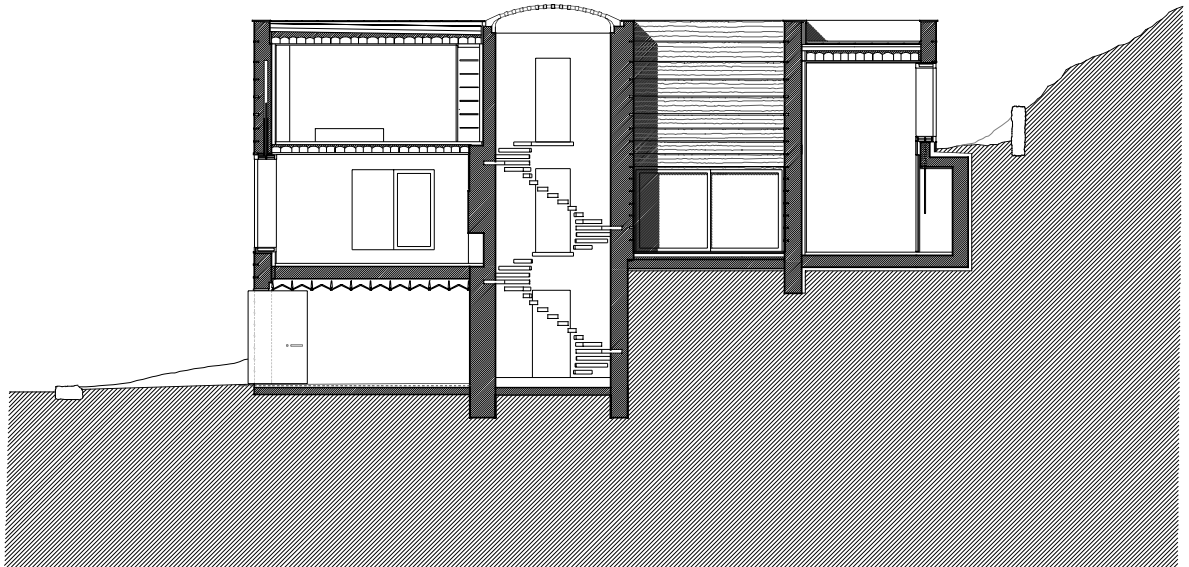
Längsschnitt C-C M 1:200
