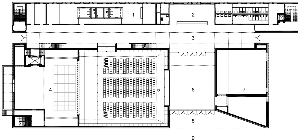
ERDGESCHOSS 0.00
