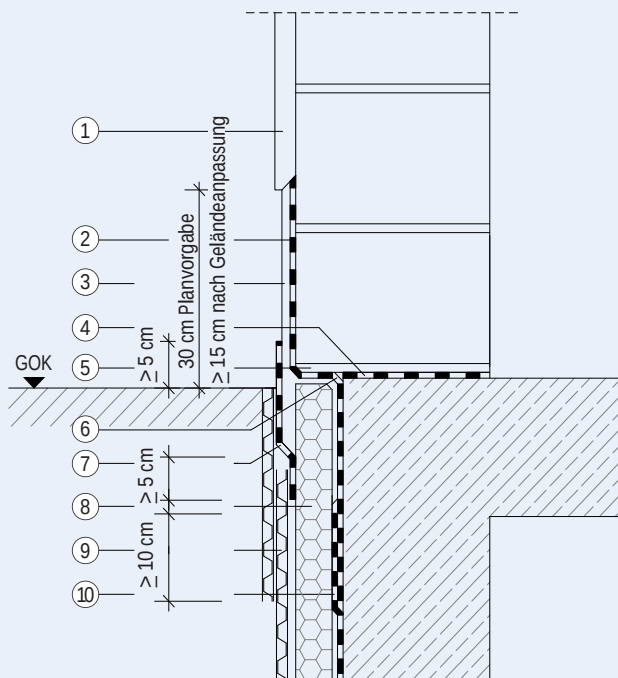
Abbildung 21: Sockelabdichtung W4-E: vorspringendes Mauerwerk mit Sockelputz
