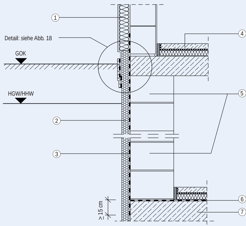
Abbildung 15: Anordnung der Abdichtung bei der Wassereinwirkung W2.1-E, Situation 2 – Übergang der PMBC-Abdichtung auf ein wasserundurchlässiges Bauteil aus Beton, Variante bündige Sohlplatte
