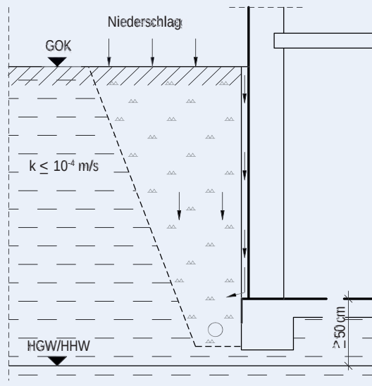
Abbildung 3: W1.2-E: Nicht drückendes Wasser bei erdberührten Wänden und Bodenplatten bei wenig durchlässigem Boden mit Dränung
