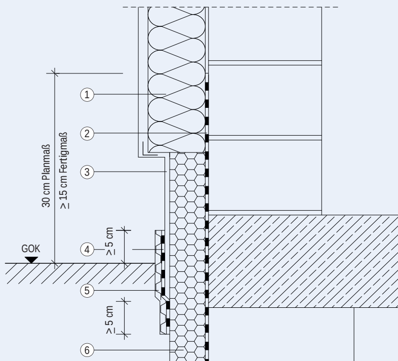
Abbildung 18: Sockelabdichtung W4-E: Wärmedämmverbundsystem (WDVS)
