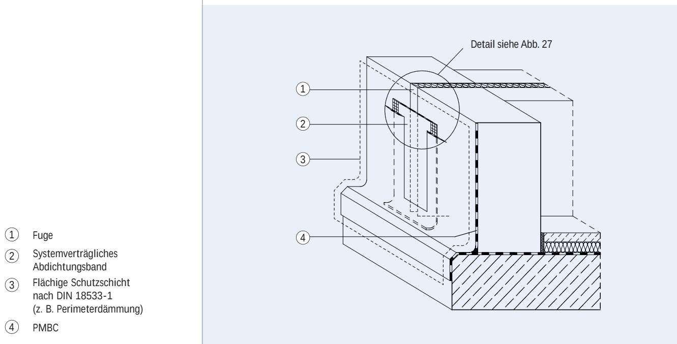
Abbildung 26: Abdichtung einer Fuge (Fugentyp I) zwischen zwei Haustrennwänden auf durchgehender Bodenplatte bei der Wassereinwirkungsklasse W1-E und W2.1-E
