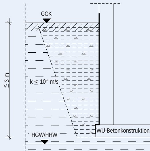
Abbildung 4: W2.1-E, Situation 1: Mäßige Einwirkung von drückendem Wasser bei Stauwasser bis 3 m Wassersäule und einer Einbindetiefe im Erdreich bis 3 m
