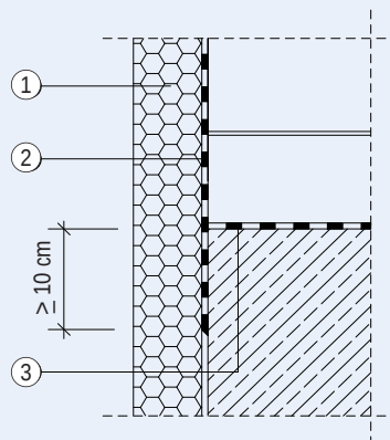
Abbildung 13: Kelleraußenwand, Fußpunkt, Variante mit bündiger Bodenplatte W 1.1-E
