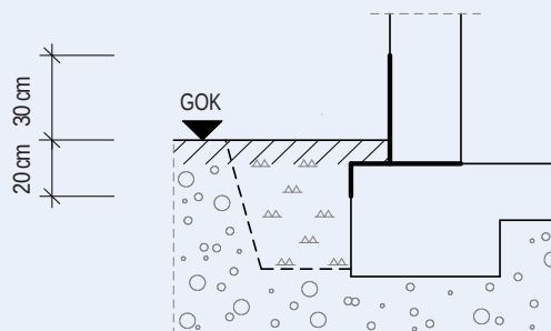
Abbildung 9: W4-E: Wassereinwirkung am Wandsockel und unter Außenwänden, nicht unterkellert
