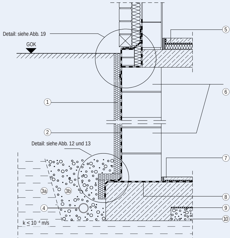
Abbildung 14: Anordnung der Abdichtung bei der Wassereinwirkungsklasse W1.2-E, Variante zweischaliges Mauerwerk
