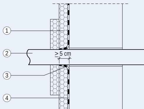
Abbildung 23: Durchdringung Kelleraußenwand bei der Wassereinwirkungsklasse W1-E
