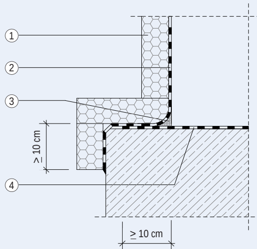
Abbildung 12: Kelleraußenwand, Fußpunkt, Variante überstehende Bodenplatte W1.1-E
