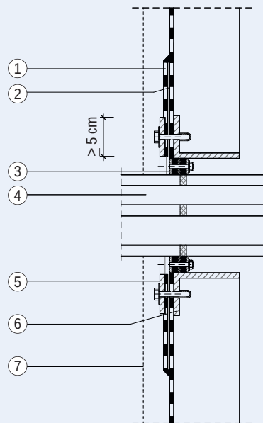
Abbildung 25: Durchdringung Kelleraußenwand mit Los- und Festflanschkonstruktion bei der Wassereinwirkungsklasse W2.1-E als Mehrspartenhauseinführung
