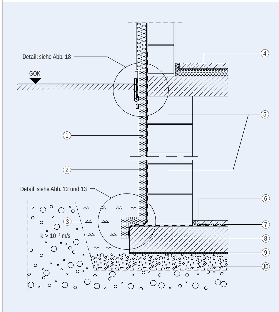
Abbildung 11: Anordnung der Abdichtung bei der Wassereinwirkung W1.1-E, Situation 2, Variante einschaliges Mauerwerk
