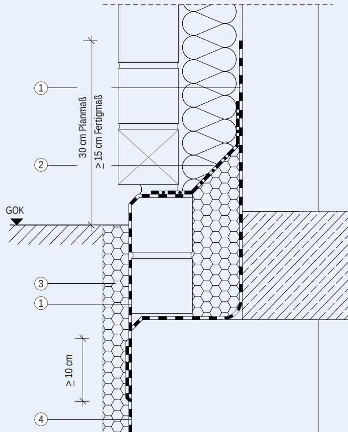
Abbildung 19: Sockelabdichtung W4-E: Fußpunktabdichtung, zweischalige Außenwand
