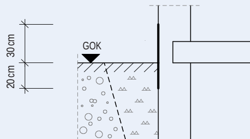
Abbildung 8: W4-E: Wassereinwirkung am Wandsockel, einschaliges Mauerwerk, unterkellert
