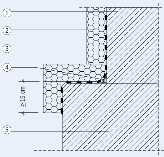
Abbildung 22: Übergänge von PMBC auf Bodenplatten aus Beton mit hohem Wassereindringwiderstand bei W2.1-E
