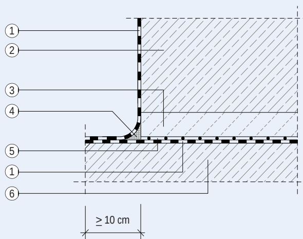
Abbildung 16: Fußpunktausbildung bei wannenförmiger Abdichtung (W2.1-E)
