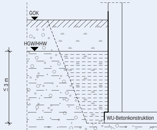
Abbildung 5: W2.1-E, Situation 2: Mäßige Einwirkung von drückendem Wasser bei Grundwasser bis 3 m Wassersäule
