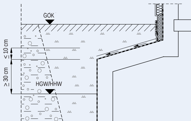
Abbildung 17: Anordnung der Abdichtung bei der Wassereinwirkungsklasse W3-E
