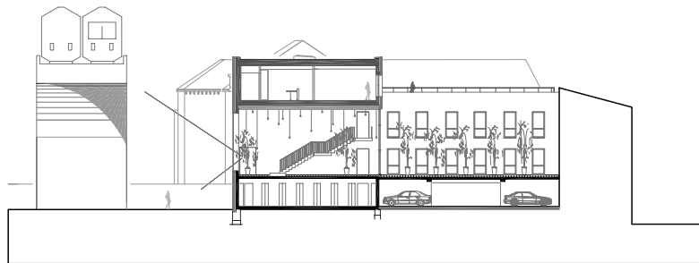
Längsschnitt durch den begrünten Innenhof
