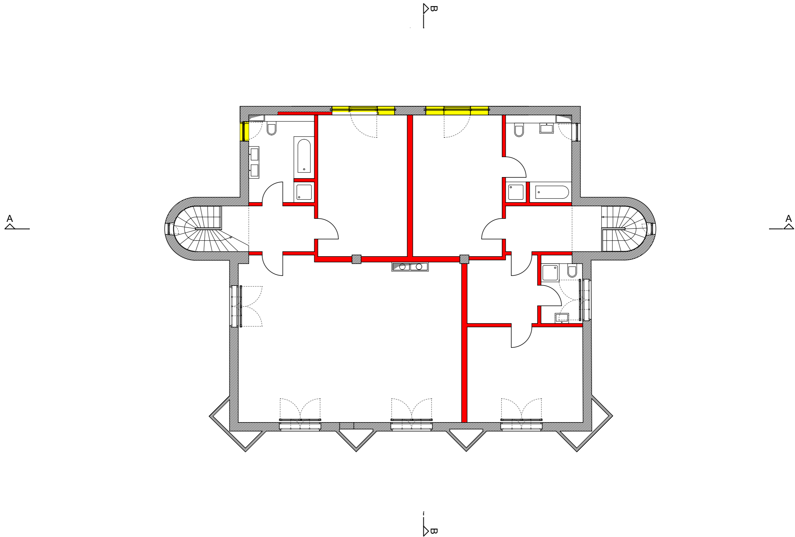
Grundriss 1. Obergeschoss M 1:100
