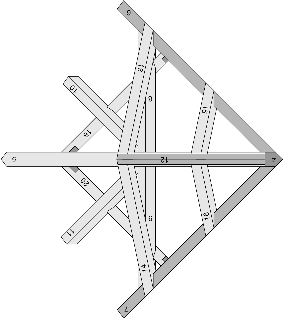
Draufsicht mit Gaube
