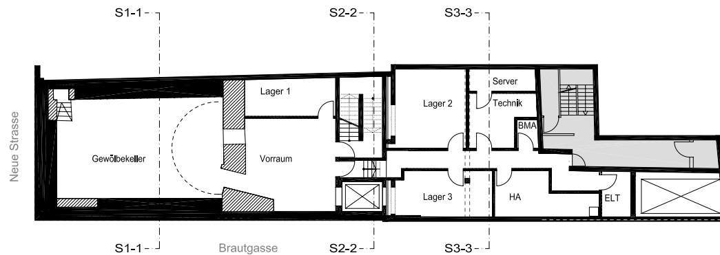
Untergeschoss
