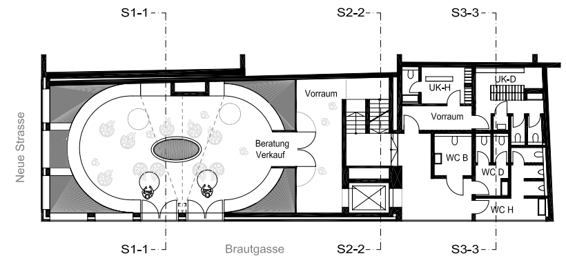
1. Obergeschoss
