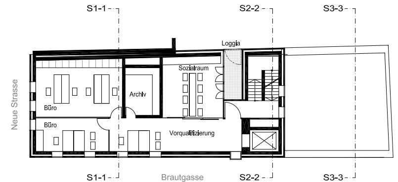
3. Obergeschoss
