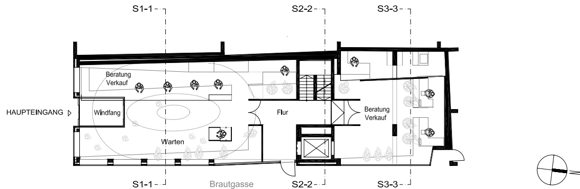
Erdgeschoss
