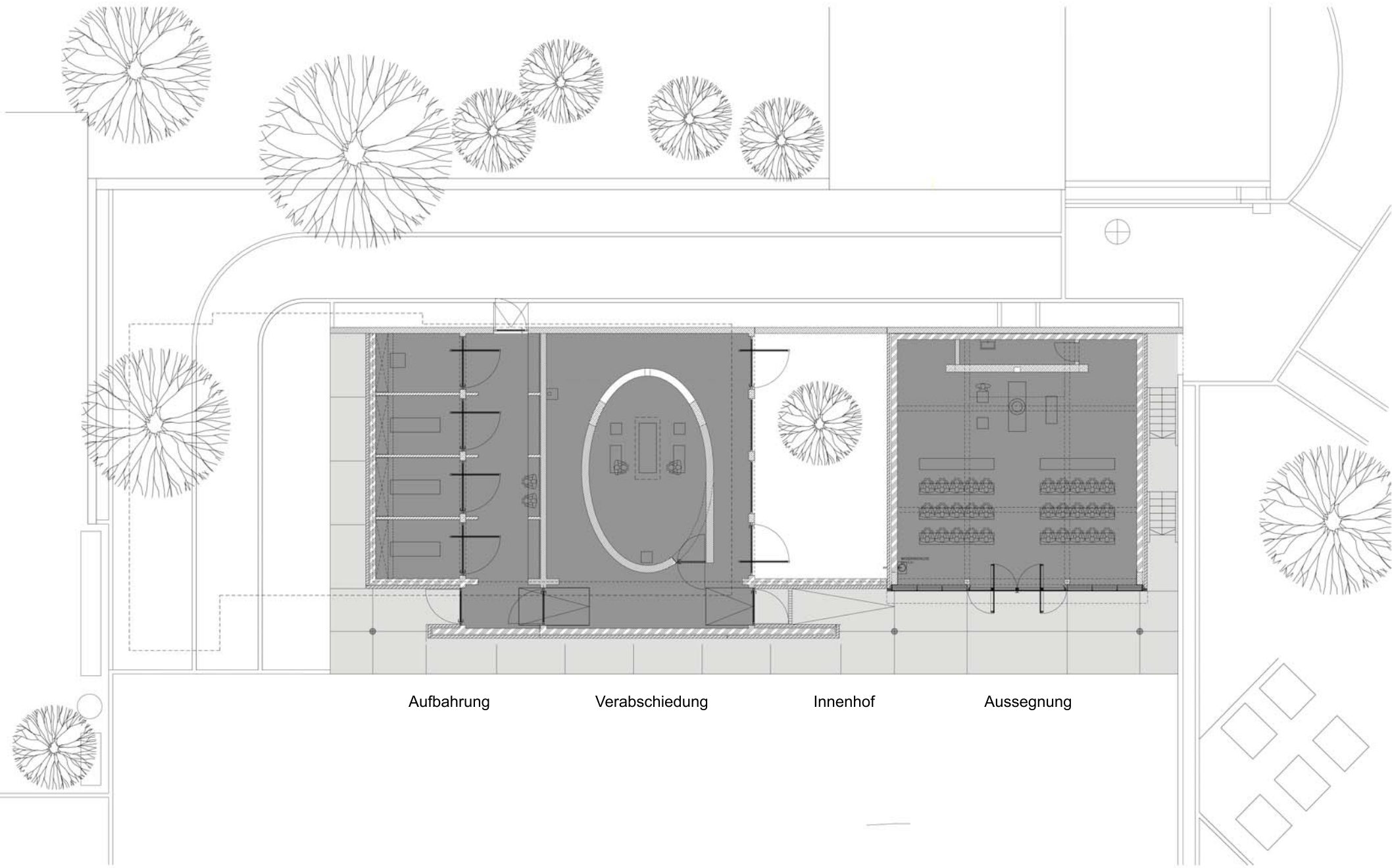
Erdgeschoss Grundriss Trauerhaus Vilsbiburg Architekt: Architekturbüro Birnkammer, Vilsbiburg
