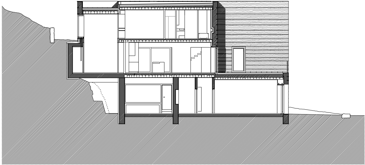
Längsschnitt A-A M 1:200
