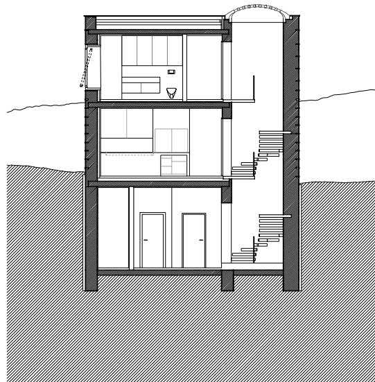
Querschnitt F-F M 1:200
