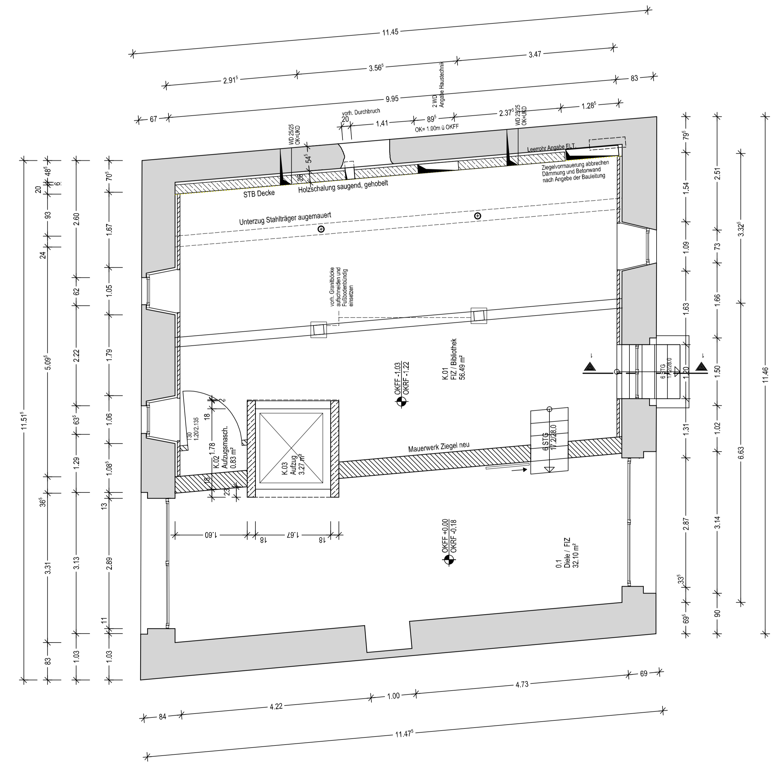
KELLERGESCHOSS
