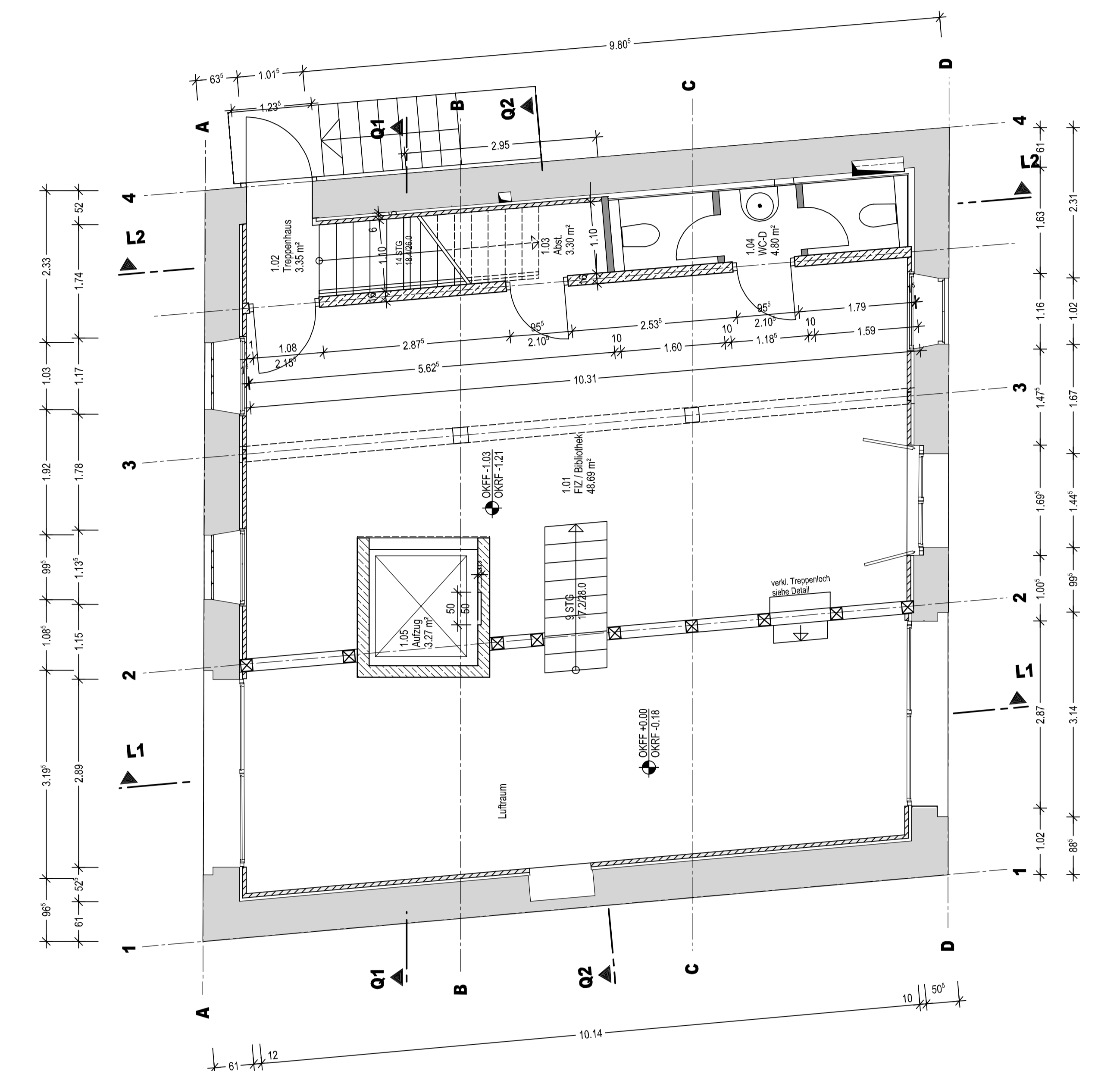
ERDGESCHOSS
