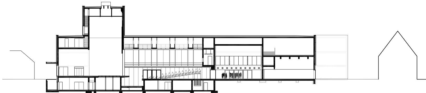
LÄNGSSCHNITT SAAL - FOYER - PROBERÄUME
