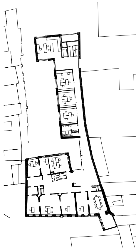
Obergeschoss
