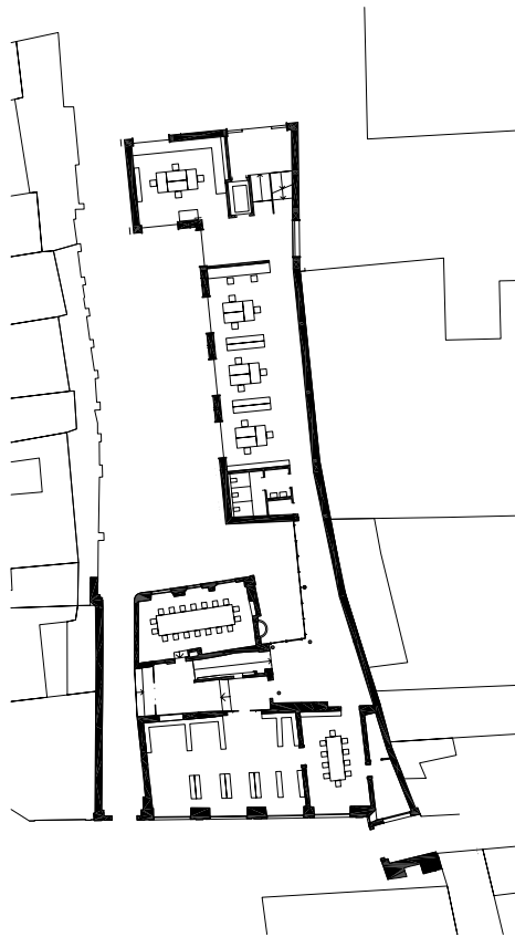
Erdgeschoss
